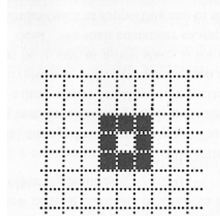
شکل ۲- سلولهای سیاه همسایه‌های سلول وسط می‌باشند
